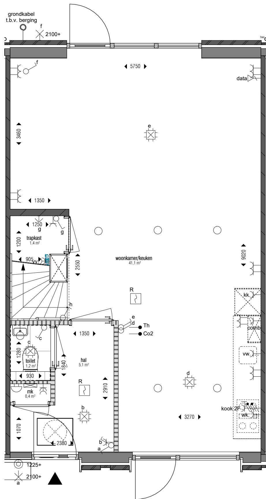
begane grond 1 : 50
