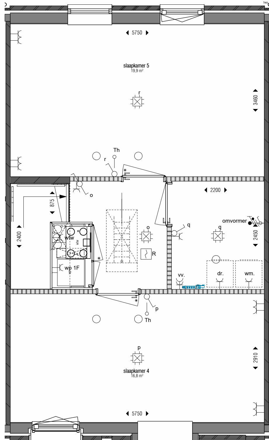
tweede verdieping 1 : 50
