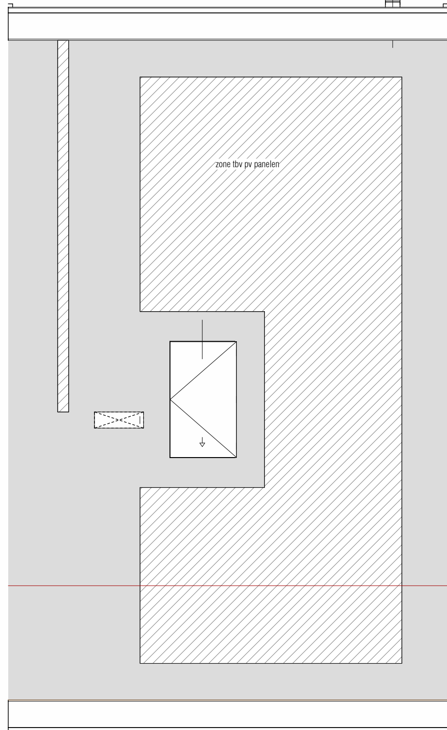
dak verdieping 1 : 50
