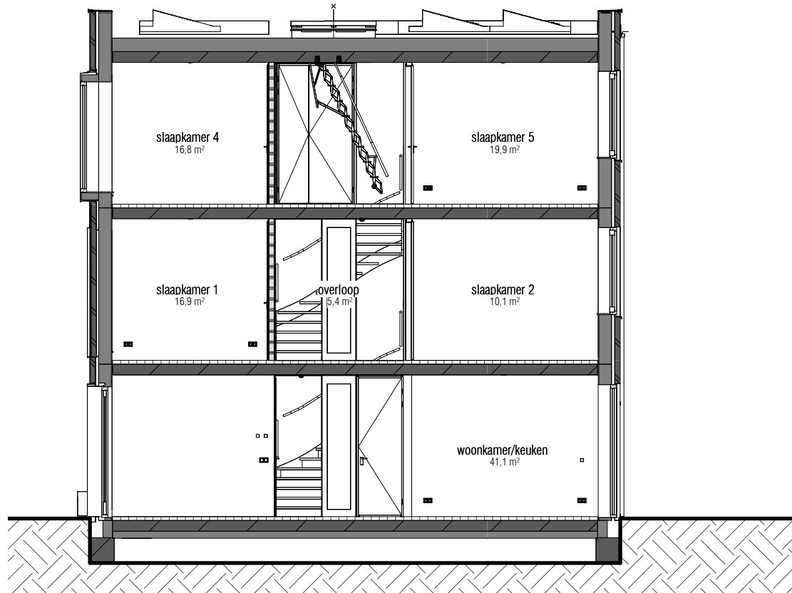
doorsnede 1 : 100
