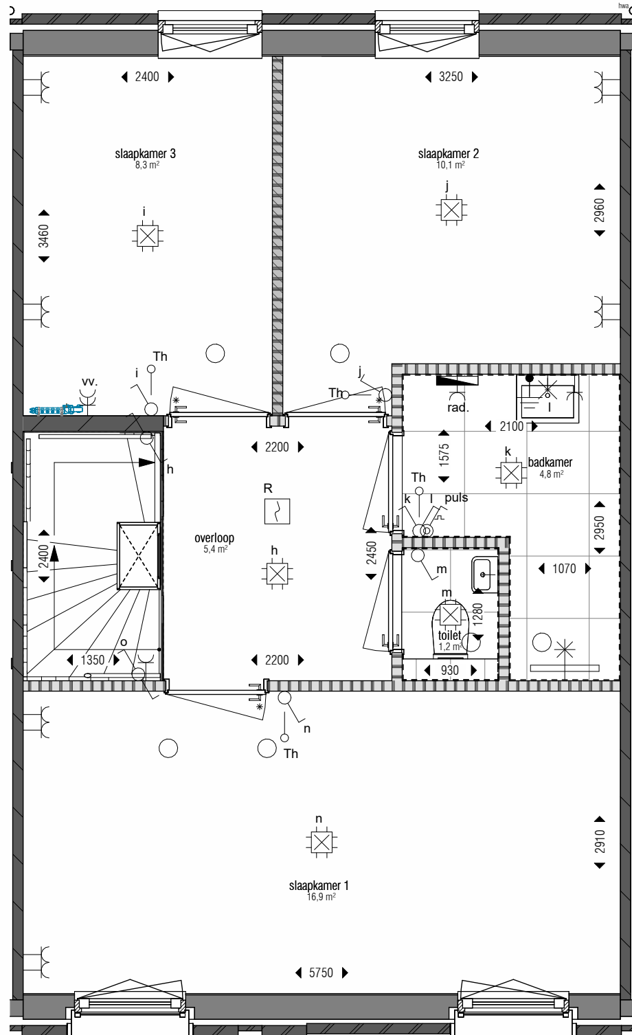
eerste verdieping 1 : 50
